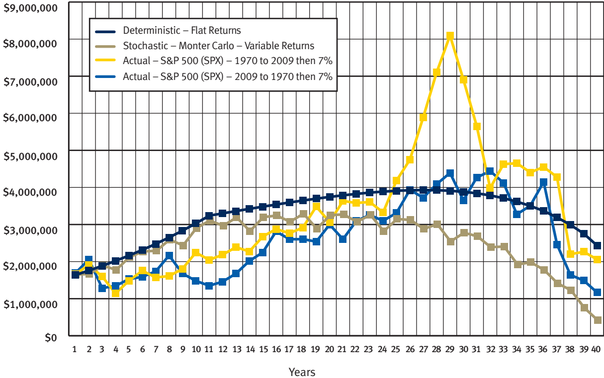
Deterministic vs. Stochastic vs. Actual Returns
